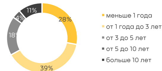
Дюрация портфеля
